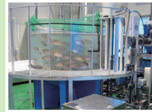
独自に開発した陸上養殖プラント
