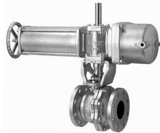
BSW型アクチュエータ付自動ボールバルブ(手動装置付)
