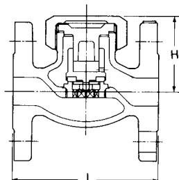
面間寸法: JIS B 2002 フランジ規格: JIS B 2239
