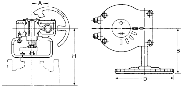
標準組み合わせおよび寸法表
