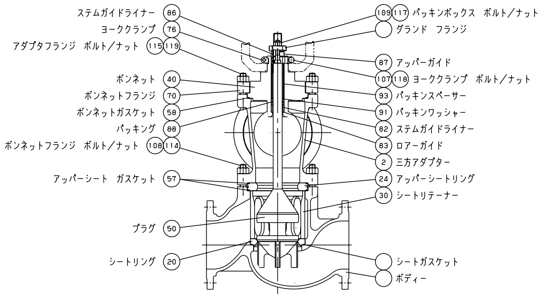
図 4. 2 三方調節弁構造図 (アダプタフランジボルトタイプ)
