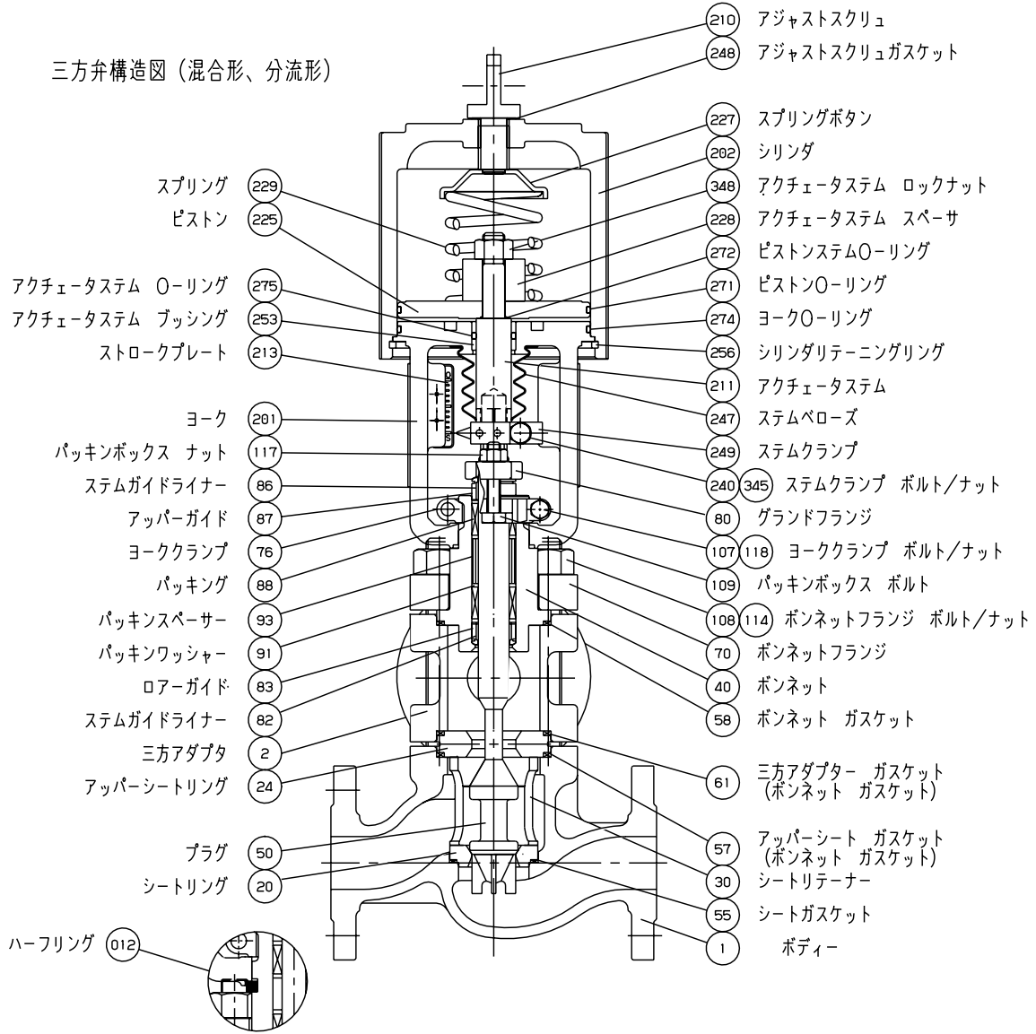
図 4. 1 三方調節弁構造図
