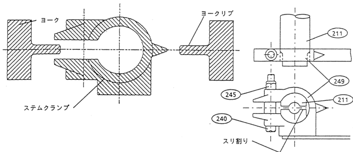
図 4. 9 アクチュエータシステムスリットとステムクランプの位置関係
