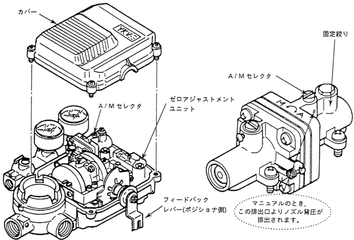
図 4. 19 A/M セレクタ
