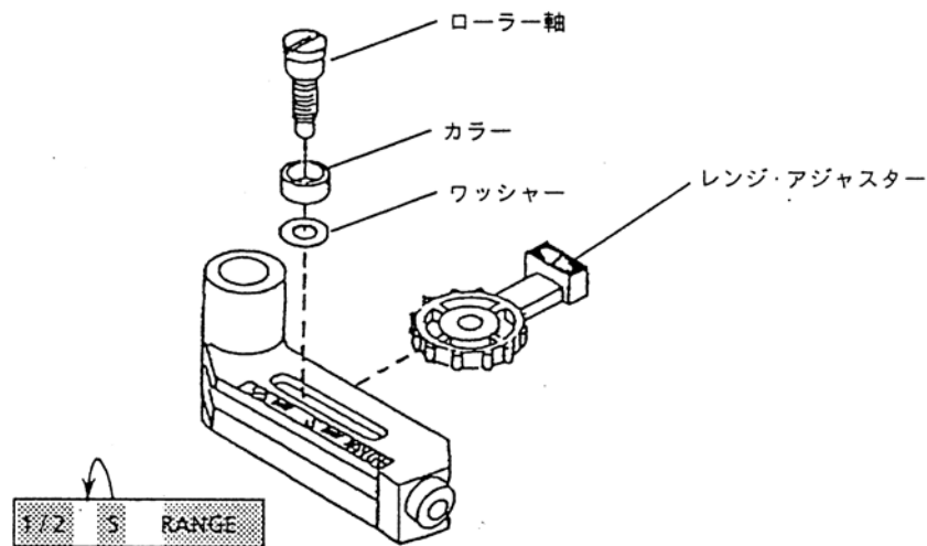
図 4. 18 スプリットレンジへの変更
