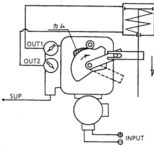
図 4. 20 入力信号とステム動作
