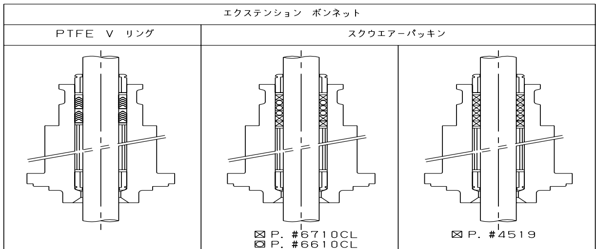
図 4. 5 エクステンションボンネット パッキン構成図
