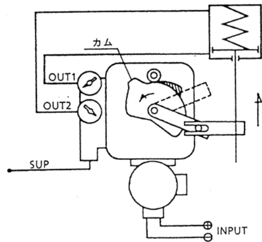
図 4. 20 入力信号とステム動作
