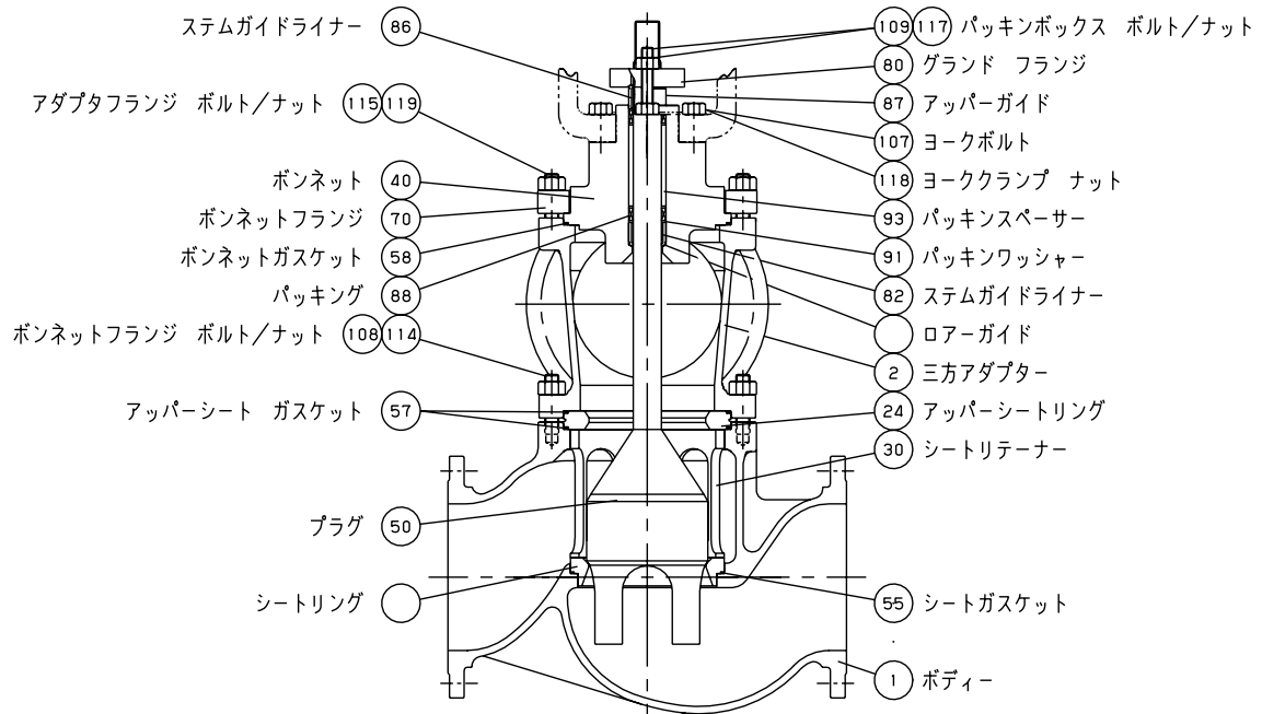
図 4. 3 三方調節弁構造図
