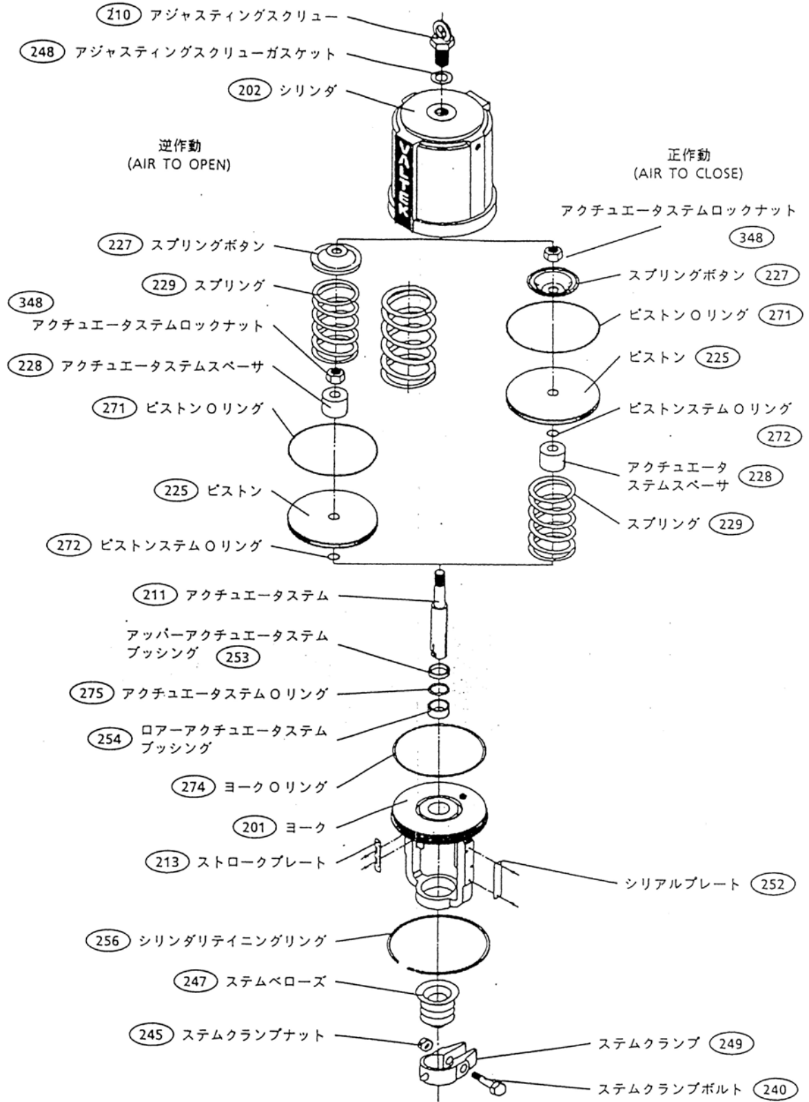
図 4. 12 アクチュエータ分解図
