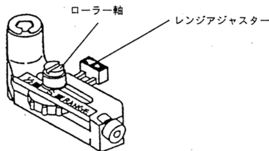
図 4.17 レンジアジャストメントユニット
