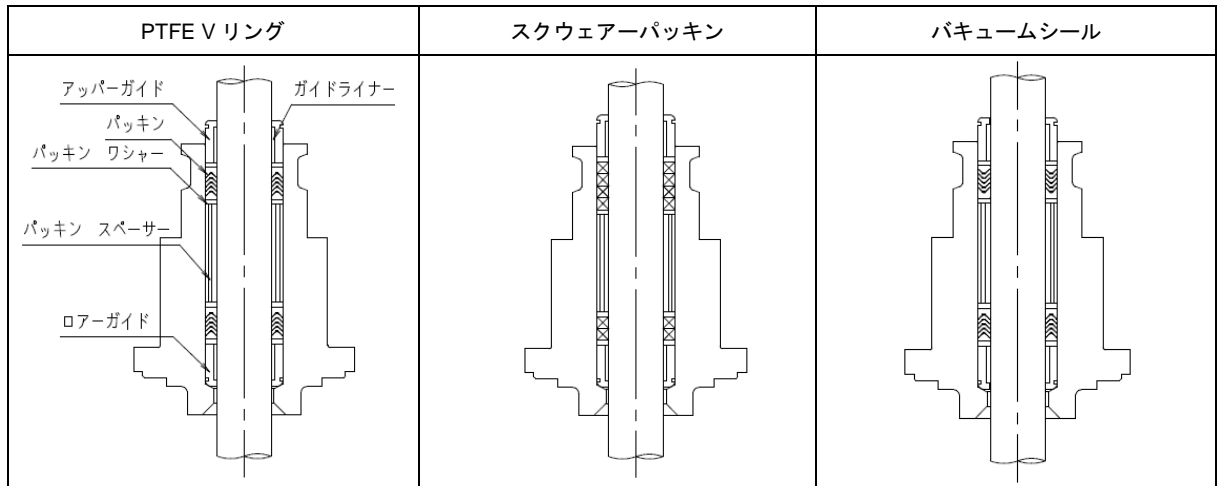
図 4. 4 標準ボンネット パッキン構成図
