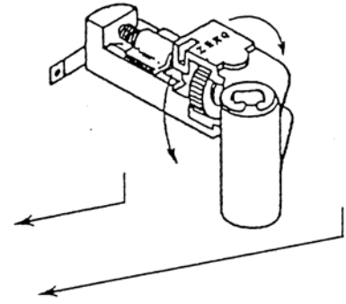
図 4. 16 ゼロアジャストメントユニット
